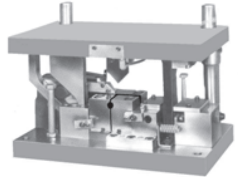
2P Cut Off Die
