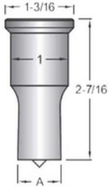
740 Punch
