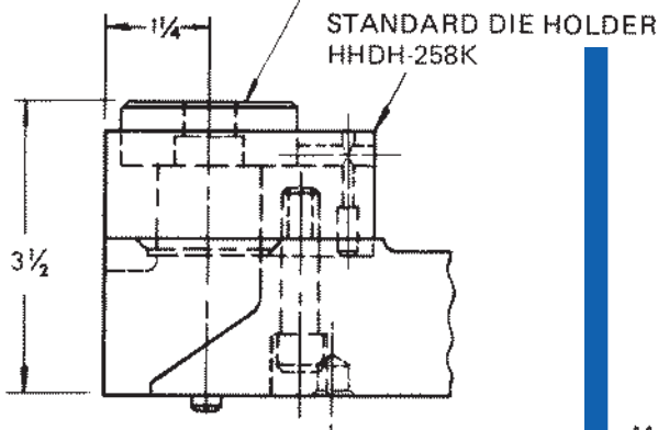
STANDARD DIE HHD-253 or HHD-253K
