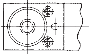
STANDARD DIE HHD-253 or HHD-253K
